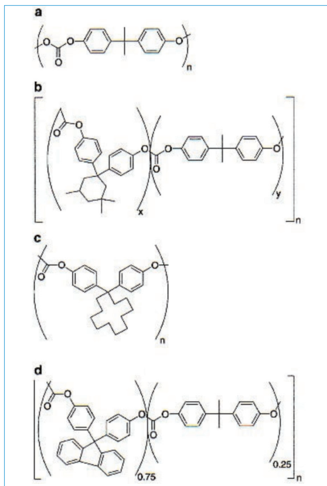
図 2: ゲストポリマーとして用いられるBisphenol A のさまざまな構造
