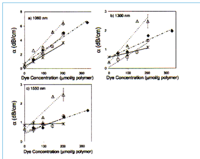
図3: 図2の4E6m/Bisphenol A polycarbonate系についてのPDS吸収損失を、3つの異なる波長で測定したものの
